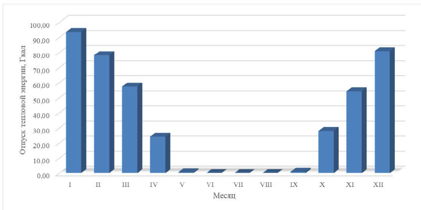
Рисунок 1.4 – Оптимальный температурный график отпуски тепловой энергии для котельной д. Тихорецкое
