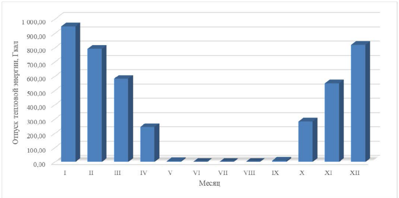
Рисунок 1.2 – Оптимальный температурный график отпуски тепловой энергии для котельной п. Новоуральский
